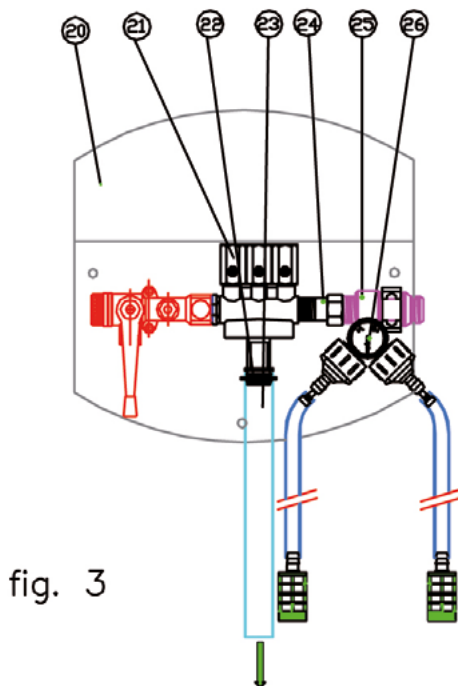
MODELE 2 PRODUITS (VERSION DISCONNECTEUR)
