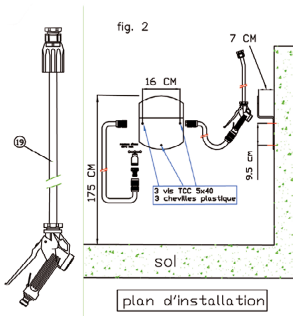
MODELE 2 PRODUITS (VERSION DISCONNECTEUR)
